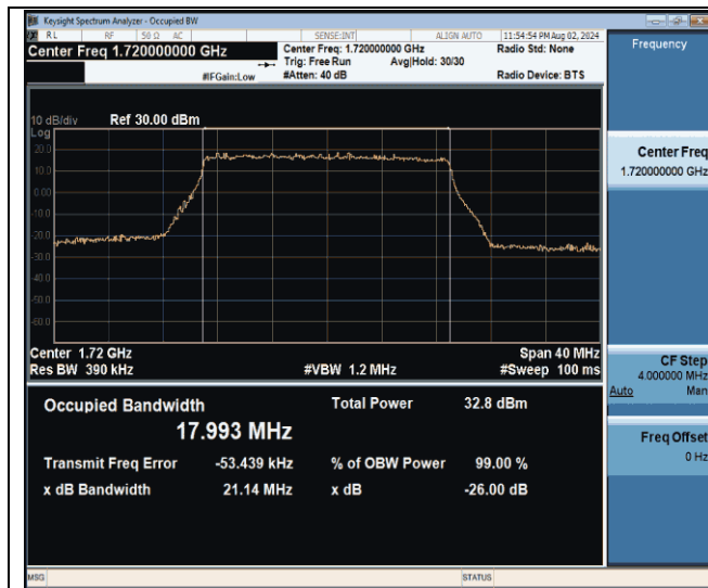
Band4-20MHz-QPSK-20050-100RB#0-PASS
