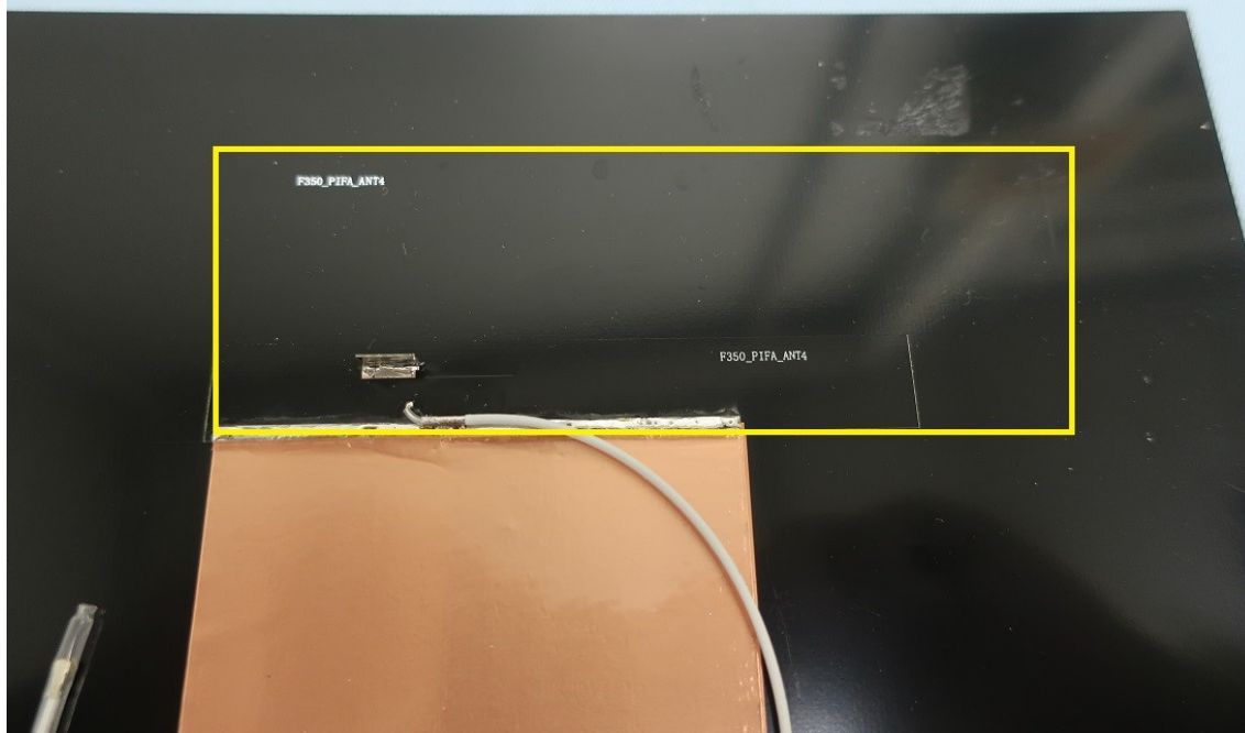
WWAN Antenna 4
