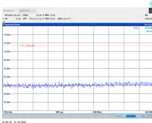
Band71-20MHz-QPSK-133222-1RB#0-Range2:0.15~30MHz
