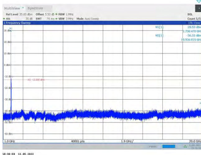
Band4-20MHz-QPSK-20300-1RB#0-Range4:1000~20000MHz
