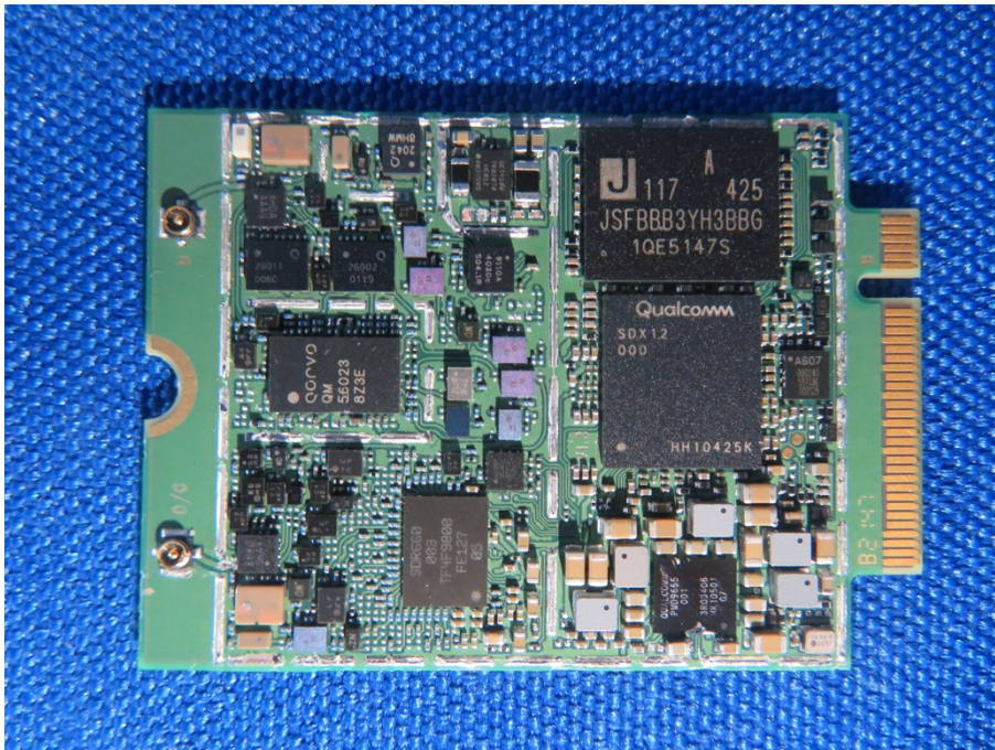
(2) EUT Photo
