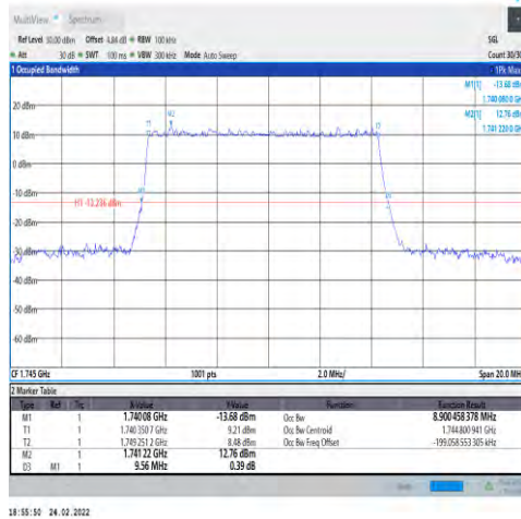
1-N66-PC3-15-10-M-1-DFT-QPSK-Outer_Ful I-50@0-Ant1-8.9-9.560-≤10-PASS
