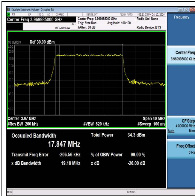
NTNV_N77-3700-3980_PC2_30_20_H_TID5_Ant1#1
