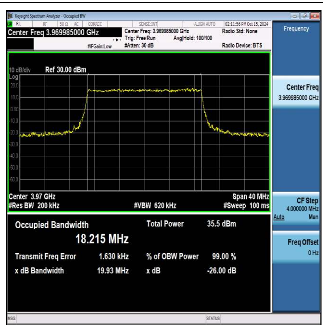
NTNV_N77-3700-3980_PC2_30_20_H_TID6_Ant1#1
