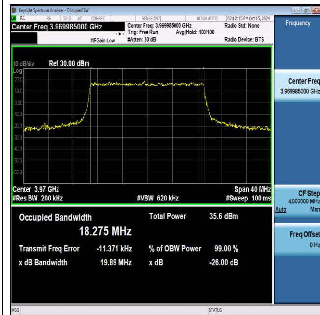
NTNV_N77-3700-3980_PC2_30_20_H_TID7_Ant1#1
