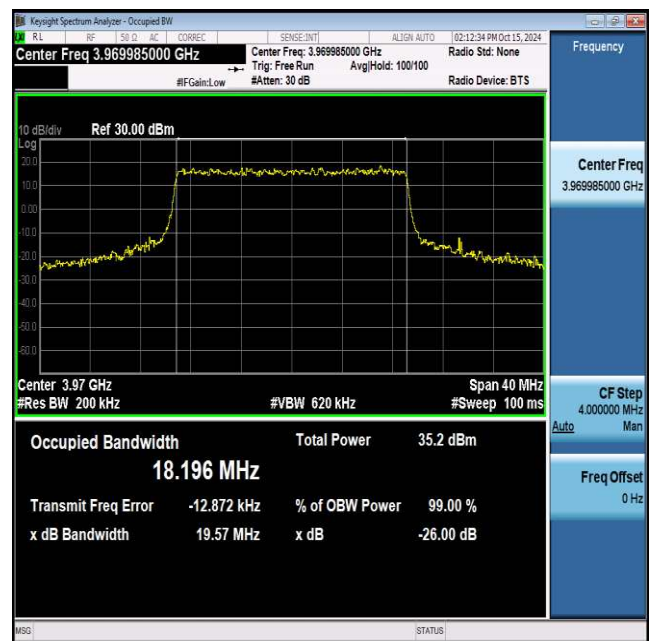
NTNV_N77-3700-3980_PC2_30_20_H_TID8_Ant1#1
