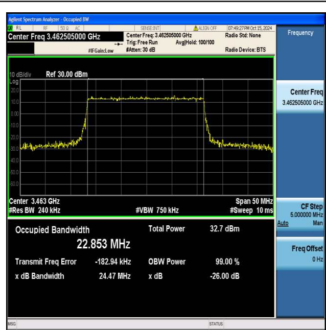
NTNV_N77-3450-3550_PC2_30_25_L_TID4_Ant1#1
