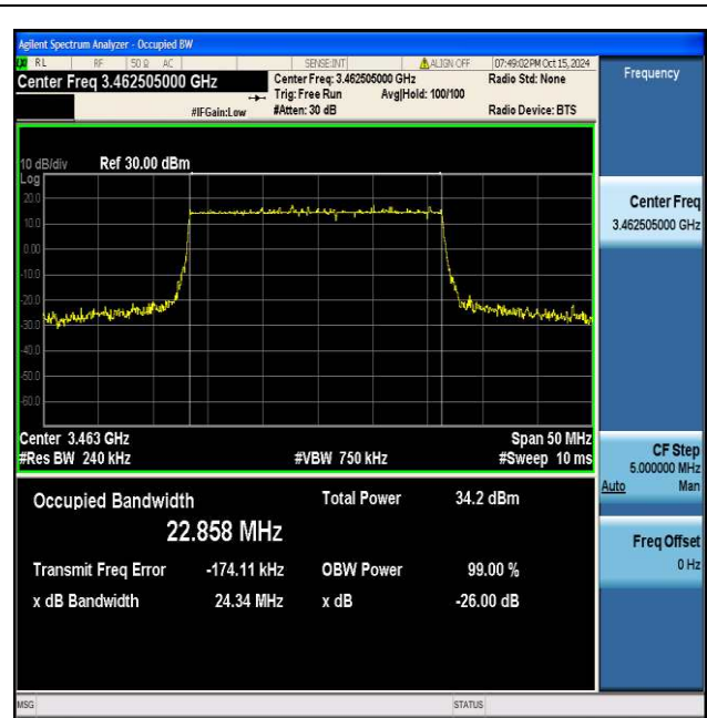
NTNV_N77-3450-3550_PC2_30_25_L_TID2_Ant1#1
