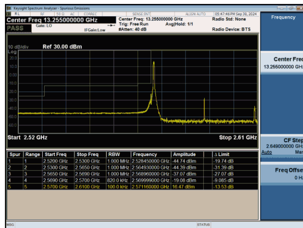
NTNV-n38-PC3-30-40-L-CP-QPSK-Edge_1RB_Left-PASS
