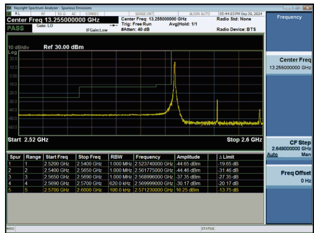
NTNV-n38-PC3-30-30-L-CP-QPSK-Edge_1RB_Left-PASS
