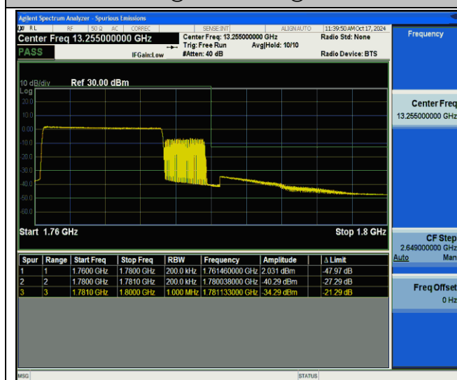
66-66-15MHz-5MHz-QPSK@QPSK-QPSK@QPSK-132549- 132642-75RB#0@75RB#0-25RB#0@25RB#0-PASS
