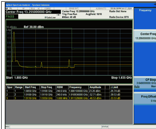
2-2-20MHz-5MHz-QPSK@QPSK-QPSK-19050-19167-1RB#0@100RB#0-0RB#0@25RB#0-PASS
