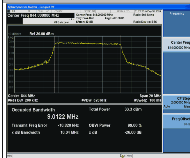
Band26(824-849)-10MHz-QPSK-26990-50RB#0-PASS
