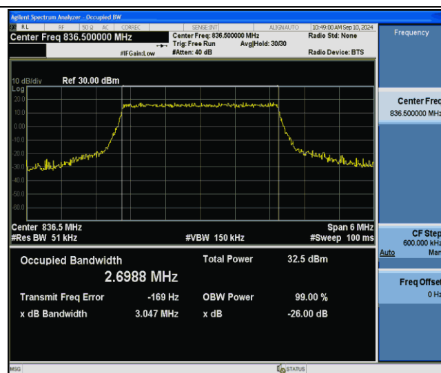
Band26(824-849)-3MHz-QPSK-26915-15RB#0-PASS
