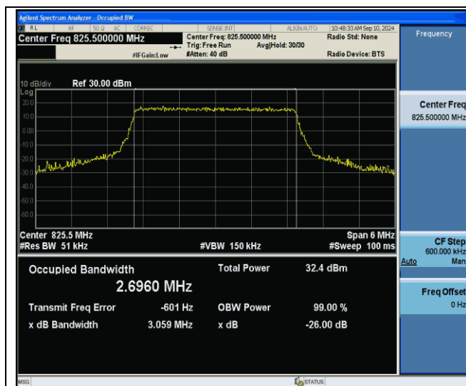
Band26(824-849)-3MHz-QPSK-26805-15RB#0-PASS
