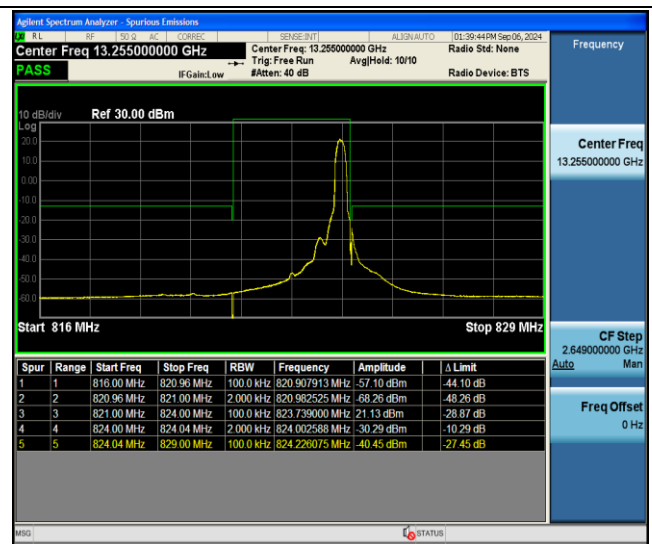
26(814-824)-3MHz-QPSK-26775-1RB#14-PASS
