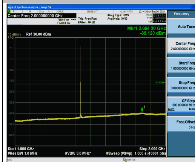
Band25-20MHz-QPSK-26365-1RB#0-1000~3000-PASS
