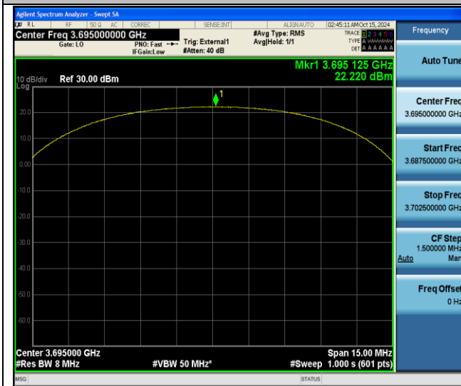
Band48-10MHz-QPSK-56690-25RB#12-PASS
