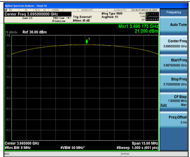
Band48-10MHz-QPSK-56690-50RB#0-PASS
