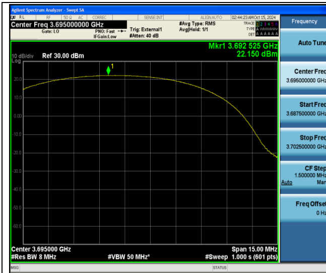
Band48-10MHz-QPSK-56690-25RB#0-PASS
