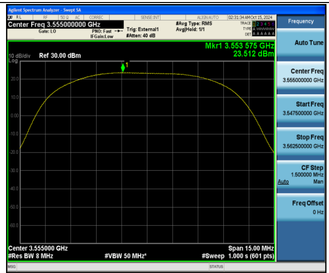
Band48-10MHz-QPSK-55290-1RB#24-PASS
