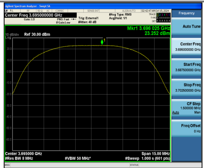
Band48-10MHz-QPSK-56690-1RB#24-PASS
