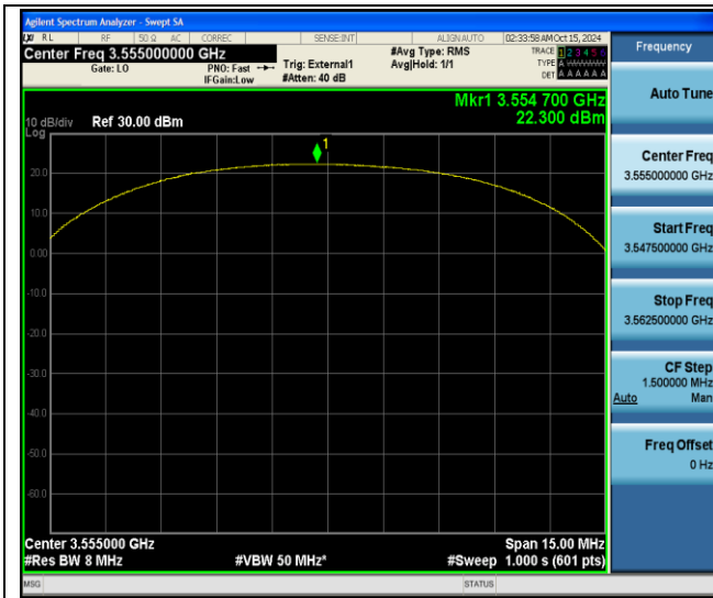
Band48-10MHz-QPSK-55290-25RB#12-PASS
