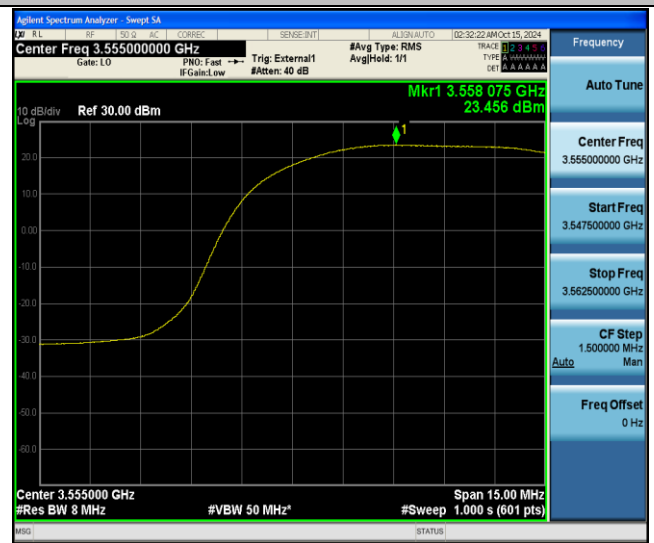
Band48-10MHz-QPSK-55290-1RB#49-PASS
