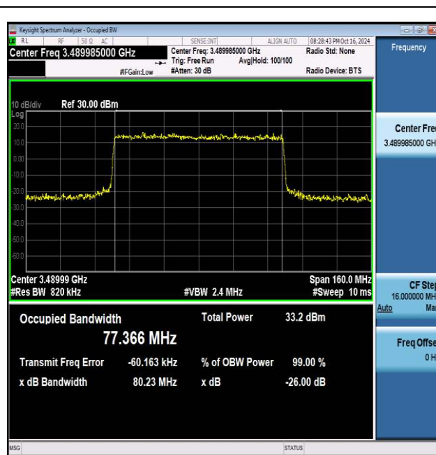
NTNV_N77-3450-3550_PC2_30_80_L_TID6_Ant1#1
