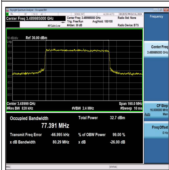
NTNV_N77-3450-3550_PC2_30_80_L_TID7_Ant1#1
