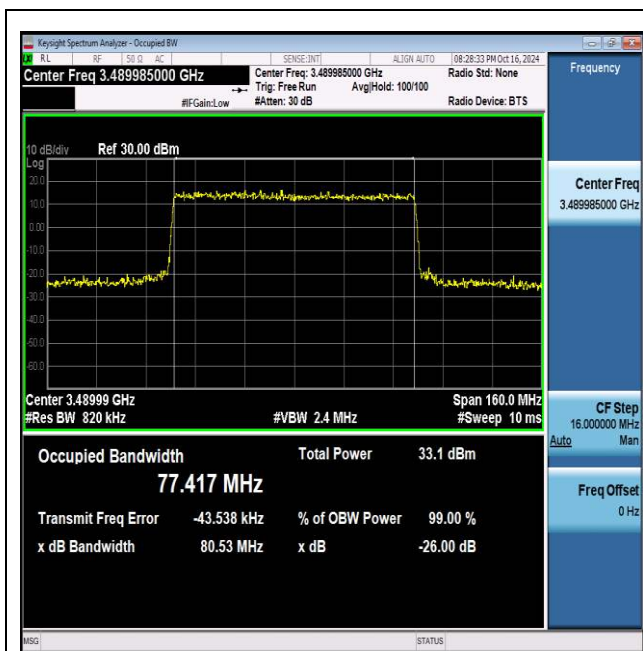
NTNV_N77-3450-3550_PC2_30_80_L_TID5_Ant1#1
