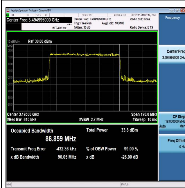
NTNV_N77-3450-3550_PC2_30_90_L_TID3_Ant1#1
