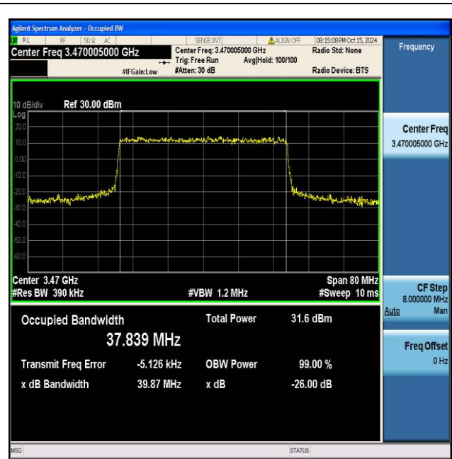
NTNV_N77-3450-3550_PC2_30_40_L_TID6_Ant1#1
