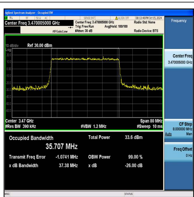
NTNV_N77-3450-3550_PC2_30_40_L_TID2_Ant1#1
