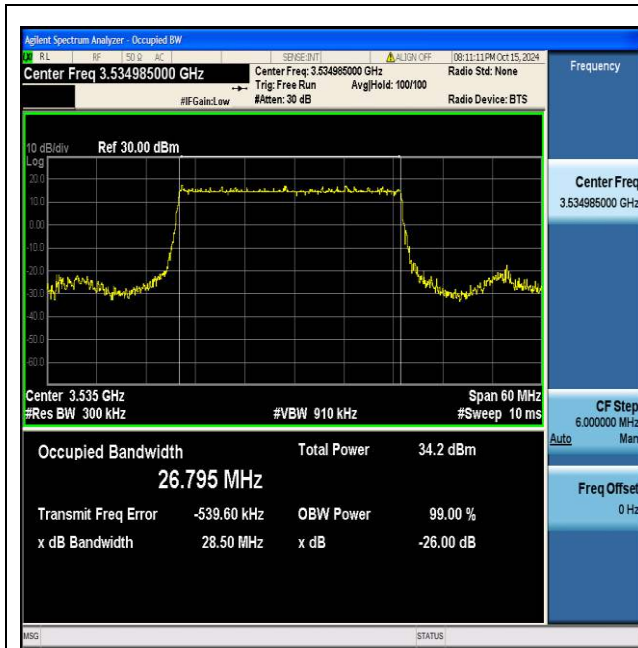
NTNV_N77-3450-3550_PC2_30_30_H_TID1_Ant1#1
