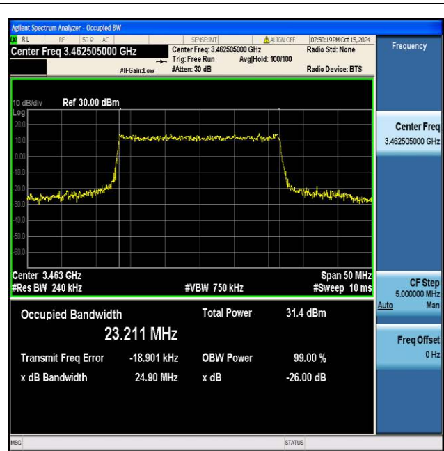
NTNV_N77-3450-3550_PC2_30_25_L_TID6_Ant1#1
