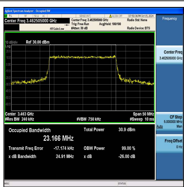
NTNV_N77-3450-3550_PC2_30_25_L_TID8_Ant1#1
