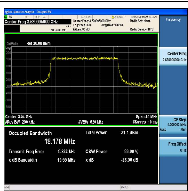
NTNV_N77-3450-3550_PC2_30_20_H_TID6_Ant1#1
