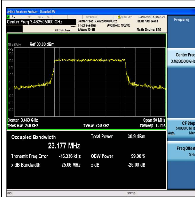
NTNV_N77-3450-3550_PC2_30_25_L_TID7_Ant1#1
