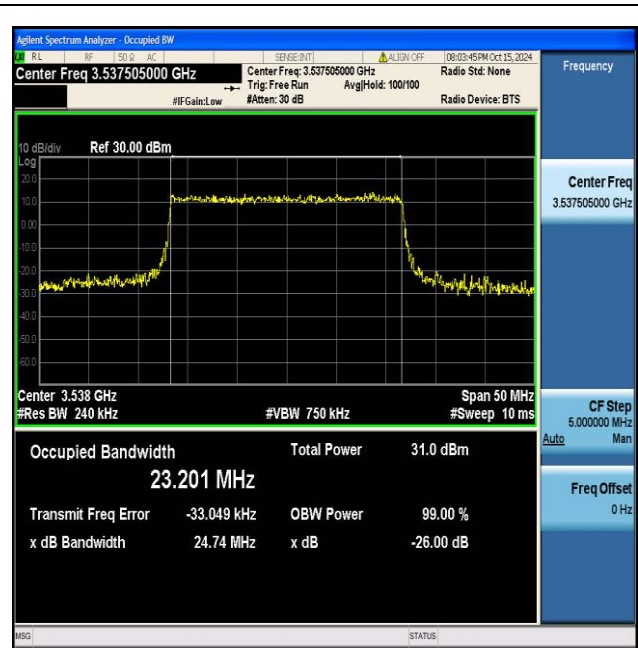
NTNV_N77-3450-3550_PC2_30_25_H_TID6_Ant1#1
