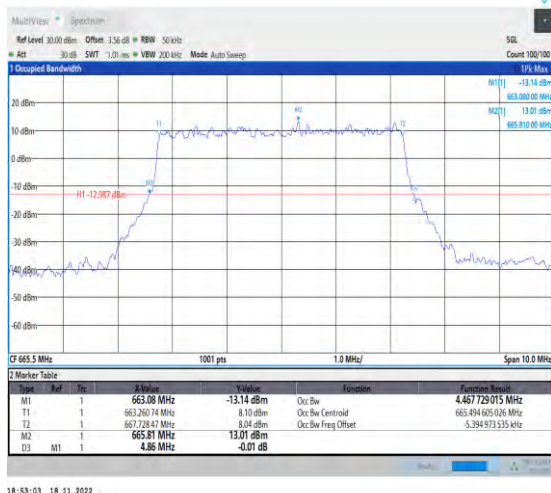
1-N71-PC3-15-5-L-1-DFT-QPSK-Outet_Full-25@0-A nt1-4.468-4.860-≤5-PASS
