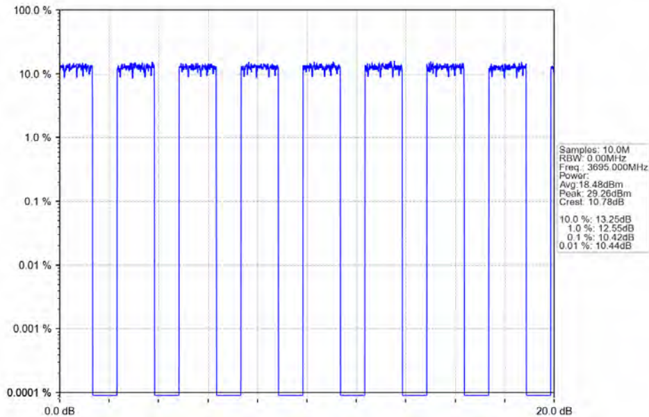
Band48_10MHz_QPSK_HCH_3695MHz_RB_50_0_NTNV
