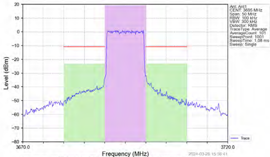
Band48_10MHz_QPSK_HCH_3695MHz_RB_50_0_NTNV
