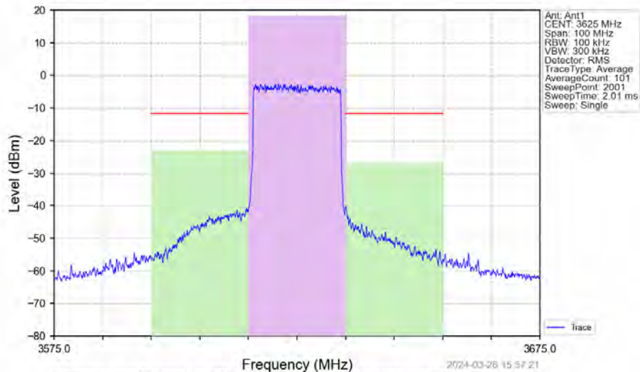
Band48_20MHz_16QAM_MCH_3625MHz_RB_100_0_NTNV
