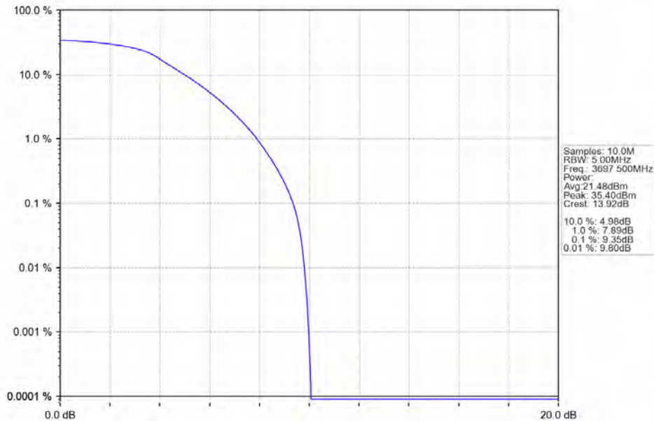
Band43c 5MHz_QPSK_HCH_3697.5MHz_RB_25_0_NTNV
