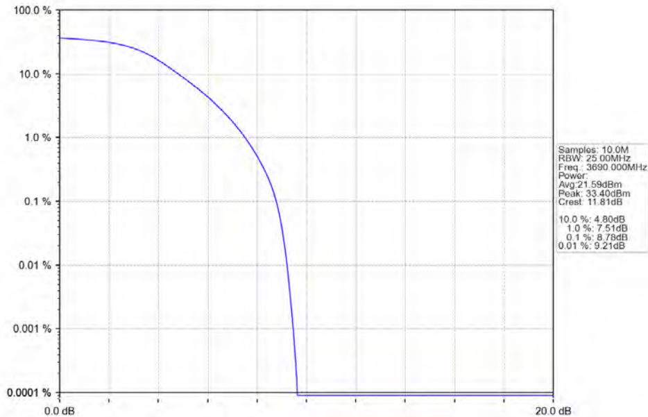
Band43c_20MHz_QPSK_HCH_3690MHz_RB_100_0_NTNV
