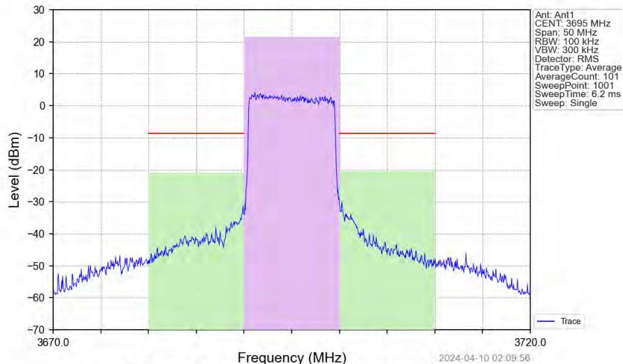
Band43c_10MHz_QPSK_HCH_3695MHz_RB_50_0_NTNV
