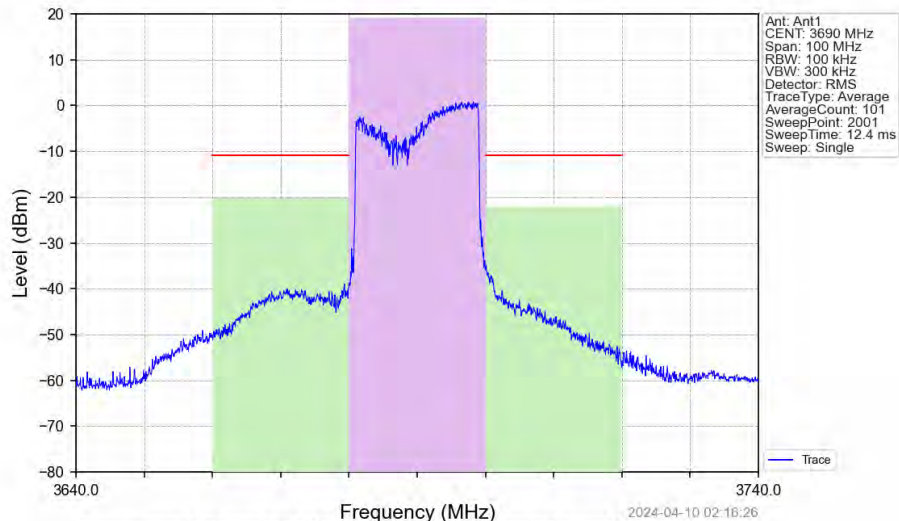
Band43c_20MHz_QPSK_HCH_3690MHz_RB_100_0_NTNV
