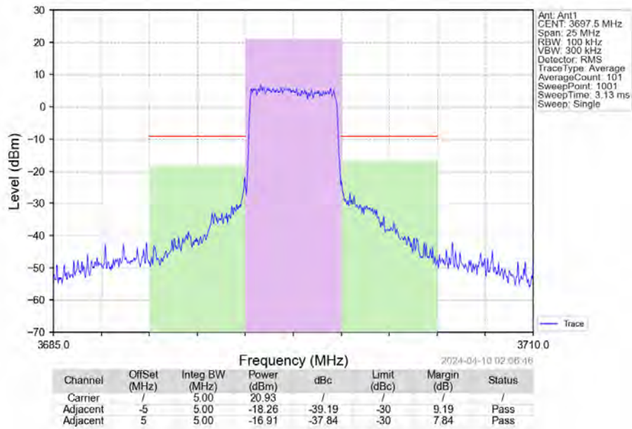
Band43c_5MHz_QPSK_HCH_3697.5MHz_RB_25_0_NTNV
