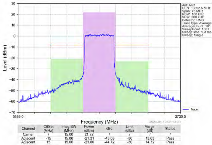
Band43c_15MHz_QPSK_HCH_3692.5MHz_RB_75_0_NTNV
