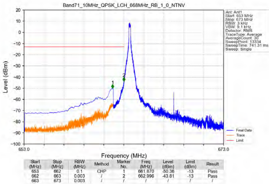
Band71_10MHz_QPSK_LCH_668MHz_RB_1_0_NTNV
