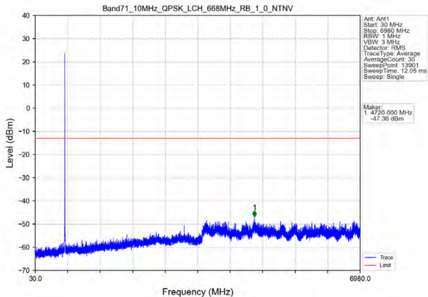
Band71_10MHz_QPSK_LCH_668MHz_RB_1_0_NTNV
