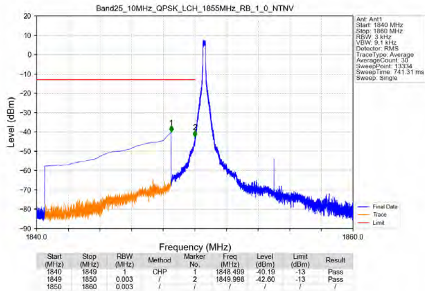
Band25_10MHz_QPSK_LCH_1855MHz_RB_1_0_NTNV
