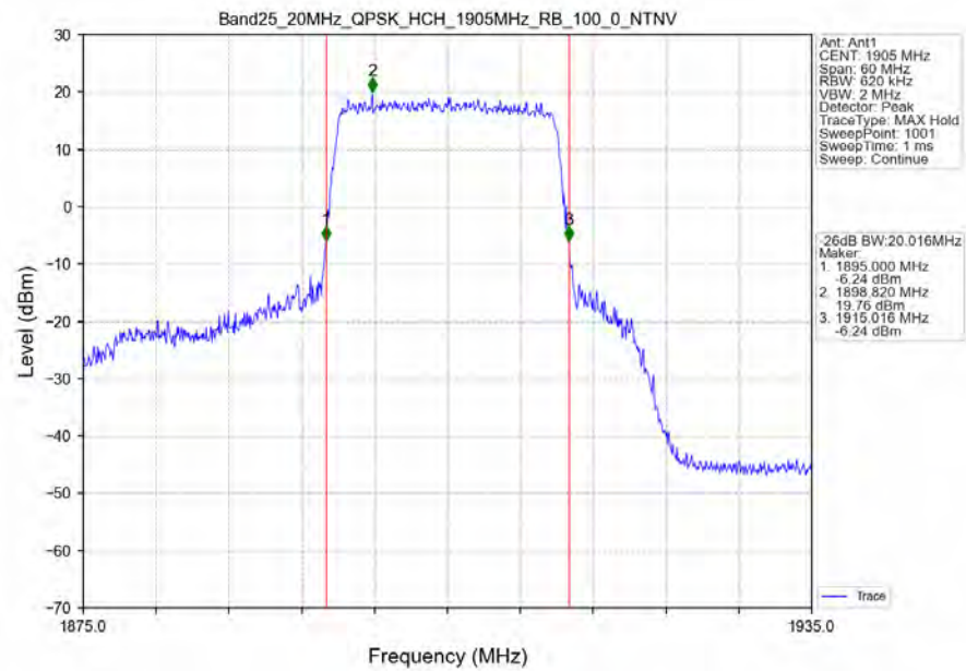
Band25_20MHz_QPSK_HCH_1905MHz_RB_100_0_NTNV
