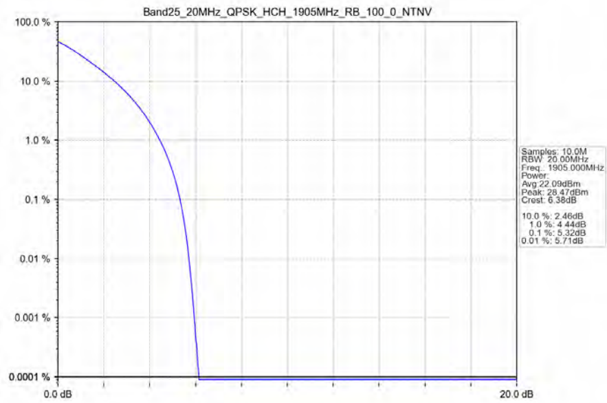
Band25_20MHz_QPSK_HCH_1905MHz_RB_100_0_NTNV
