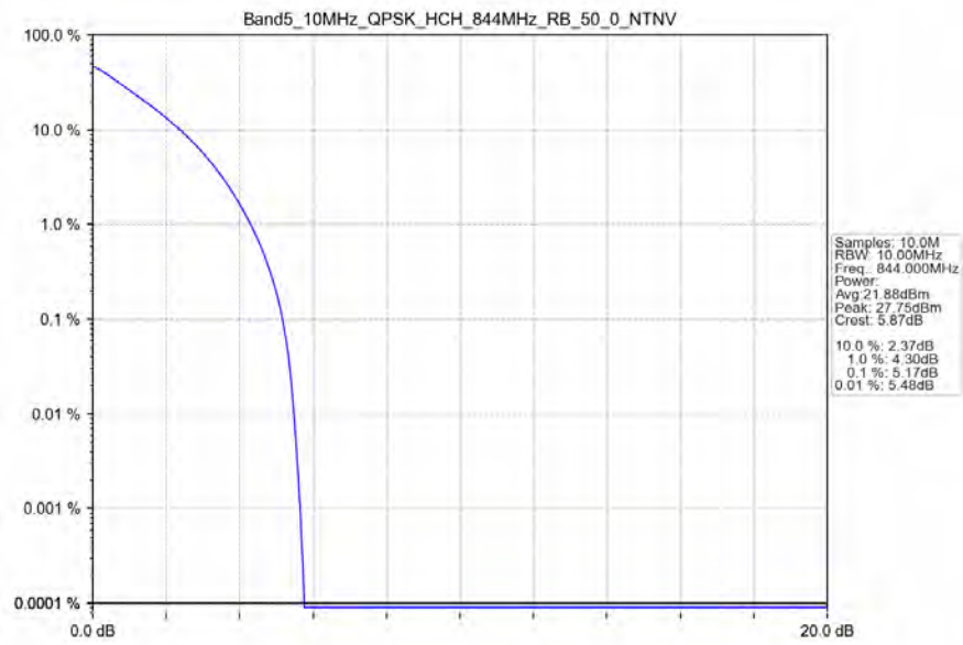
Band5_10MHz_QPSK_HCH_844MHz_RB_50_0_NTNV
