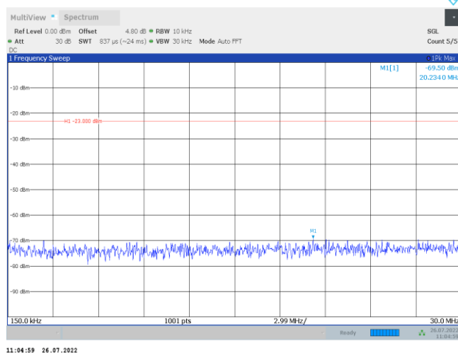
Band25-5MHz-QPSK-26065-1RB#0-Range2:0.15~30MHz
