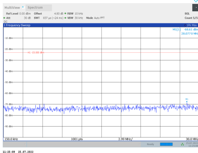
Band4-20MHz-QPSK-19975-1RB#0-Range2:0.15~30MHz
