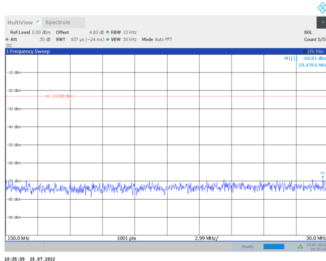
Band2-5MHz-QPSK-18700-1RB#0-Range2:0.15~30MHz
