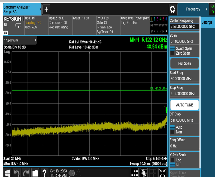
11AX40MIMO_Ant2_5270_30~5140
