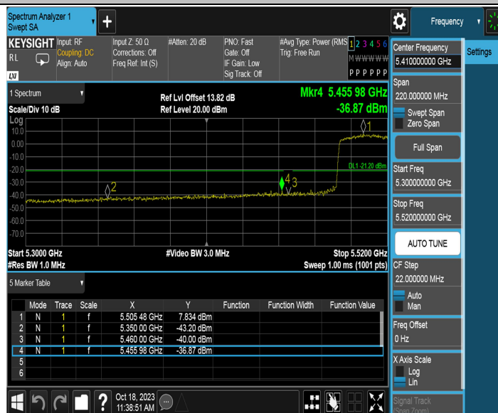
11AX40MIMO_Ant1_Low_5510_Peak
