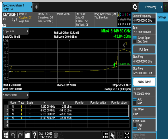
11AX80MIMO_Ant2_Low_5210_Peak
