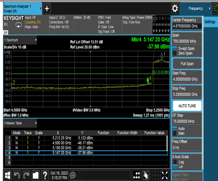
11AX80MIMO_Ant2_Low_5210_AV
