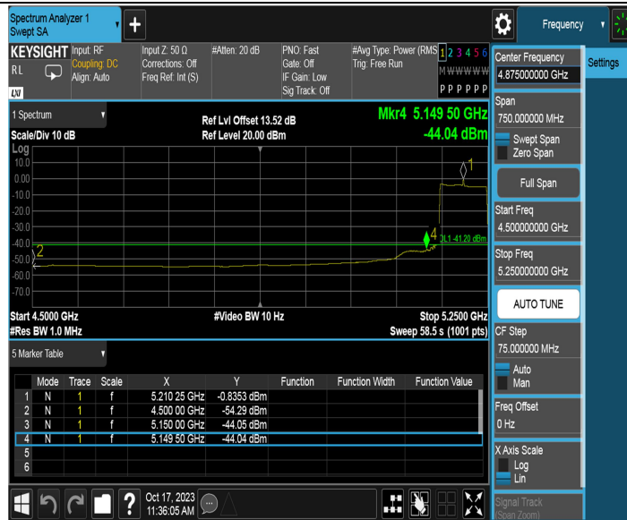
11AC80MIMO_Ant2_Low_5210_Peak
