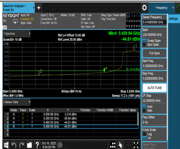
11AC40MIMO_Ant2_Low_5510_AV
