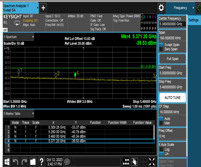
11N40MIMO_Ant2_High_5310_AV
