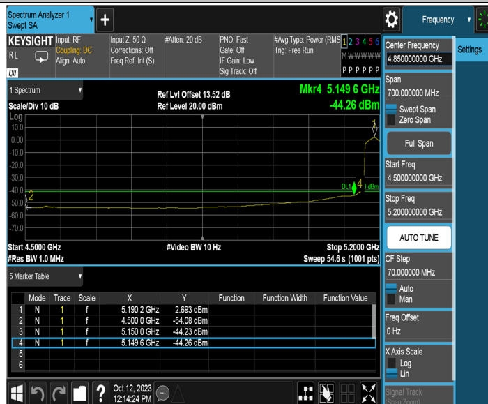
11N40MIMO_Ant2_Low_5190_AV
