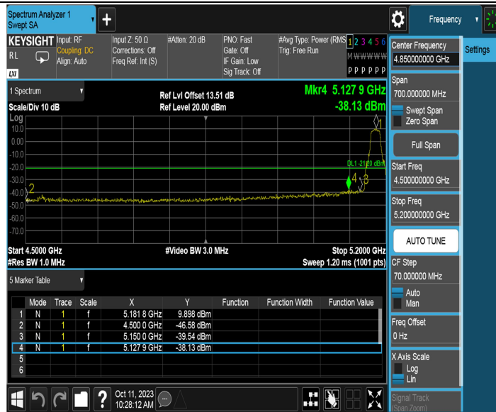
11N20MIMO_Ant2_Low_5180_AV
