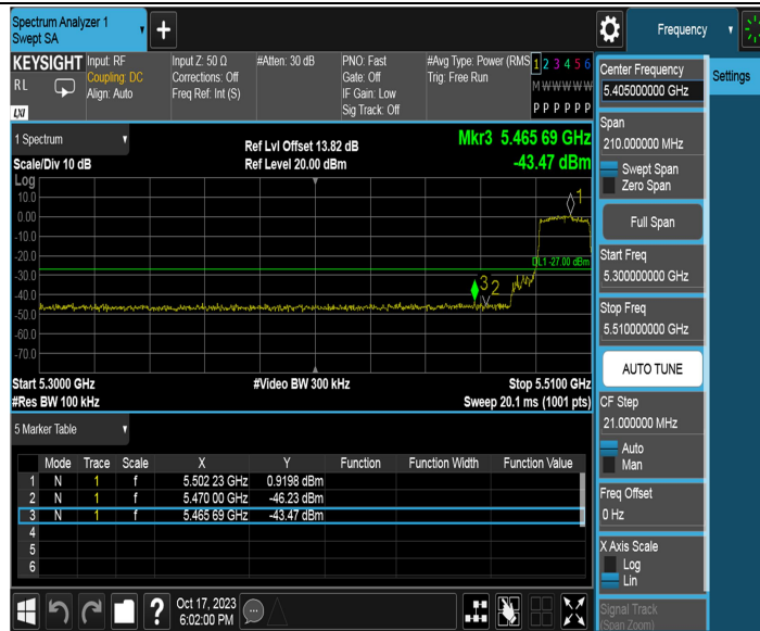
11AX20MIMO_Ant2_Low_5500
