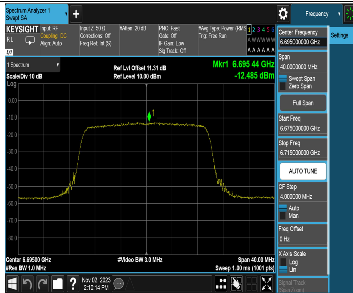
11AX20MIMO_Ant2_6695
