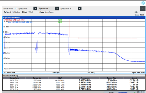
41-41-20MHz-20MHz-QPSK-QPSK-41292-4149 0-1RB#99-1RB#0
