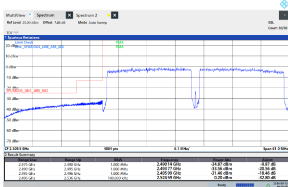
41-41-20MHz-20MHz-QPSK-QPSK-39750-39948-1RB #99-1RB#0
