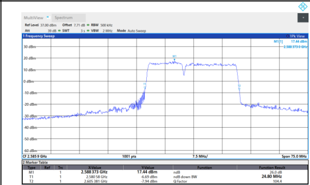
41-41-10MHz-20MHz-QPSK-QPSK-39705-39849-50R B#0-100RB#0
