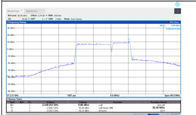
7-7-20MHz-10MHz-QPSK-QPSK-21251-21395-100RB #0-50RB#0
