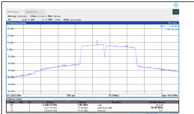
7-7-20MHz-10MHz-QPSK-QPSK-20850-20994-100RB #0-50RB#0
