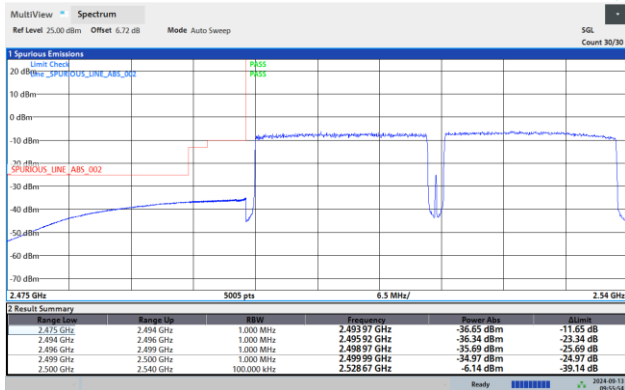
7-7-20MHz-20MHz-QPSK-QPSK-20850-21048-21048-1R B#99-1RB#0
