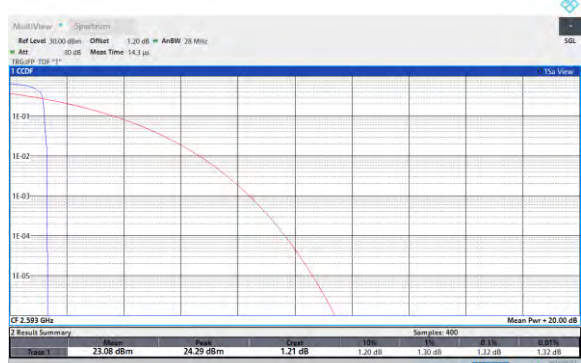
Band41-20MHz-64QAM-41490-1RB#0
