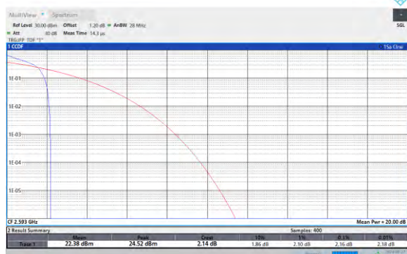
Band41-20MHz-QPSK-41490-1RB#0
