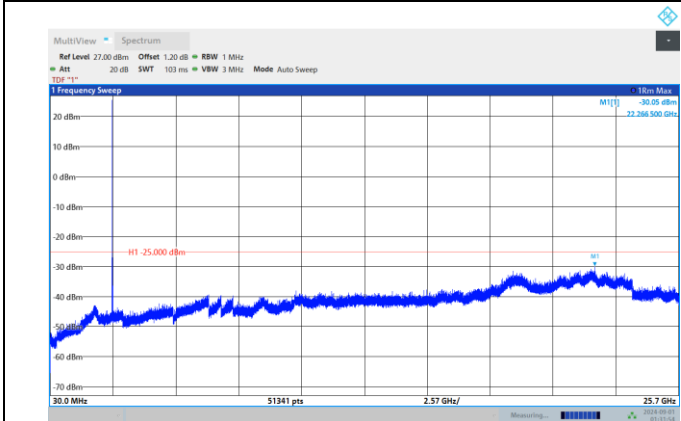
Band7-20MHz-QPSK-21100-1RB#0-Range:30~25700MH Z
