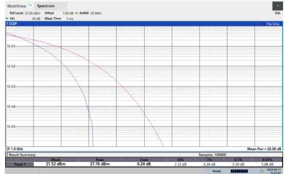
Band2-20MHz-16QAM-18700-100RB#0
