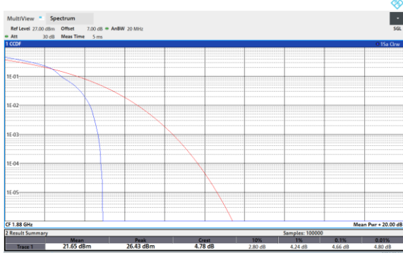
Band2-20MHz-16QAM-19100-1RB#0
