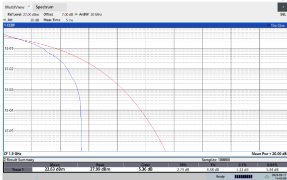
Band2-20MHz-16QAM-18700-1RB#0
