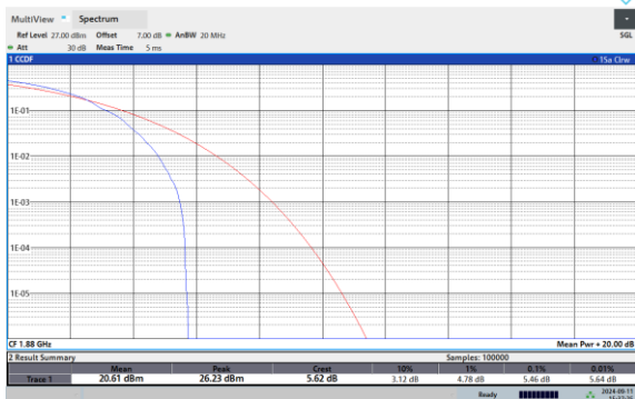
Band2-20MHz-64QAM-19100-1RB#0
