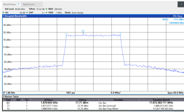
Band2-20MHz-16QAM-18700-100RB#0
