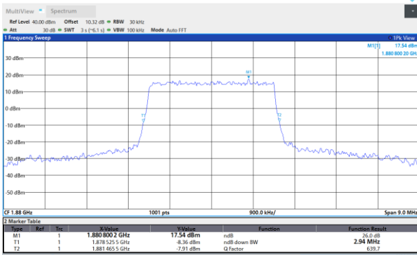
Band2-3MHz-16QAM-18615-15RB#0
