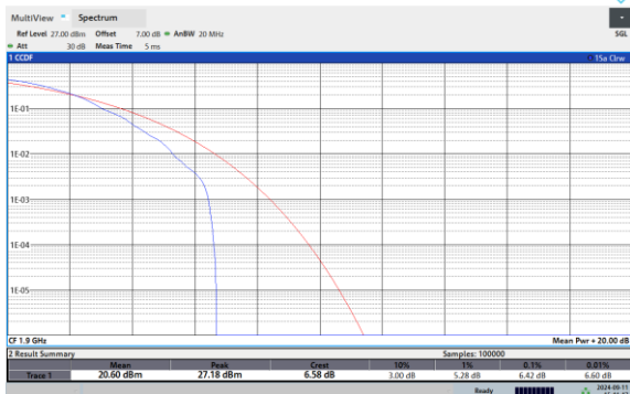
Band2-20MHz-64QAM-19100-1RB#0
