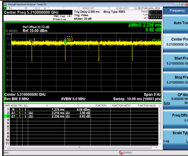
11AX80MIMO Ant9 5210
