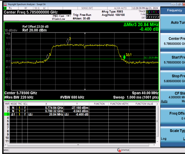
11N20MIMO Ant9 5785
