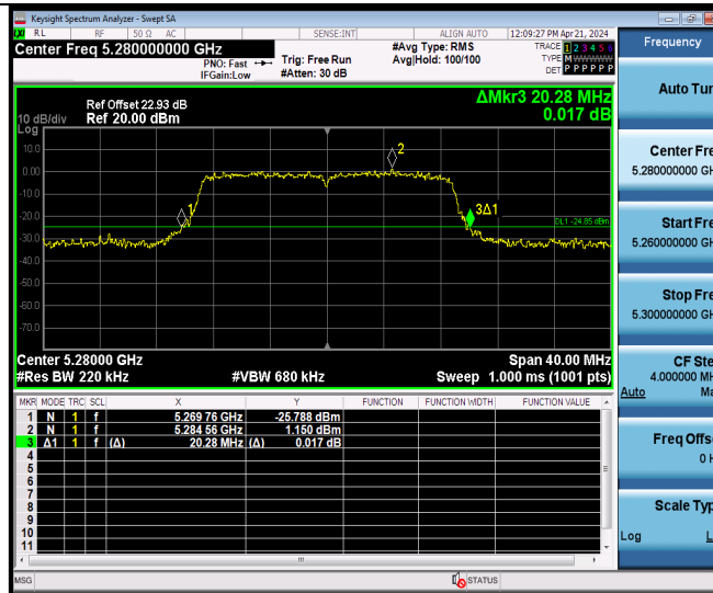
11N20MIMO Ant9 5280
