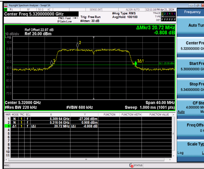
11N20MIMO Ant9 5320
