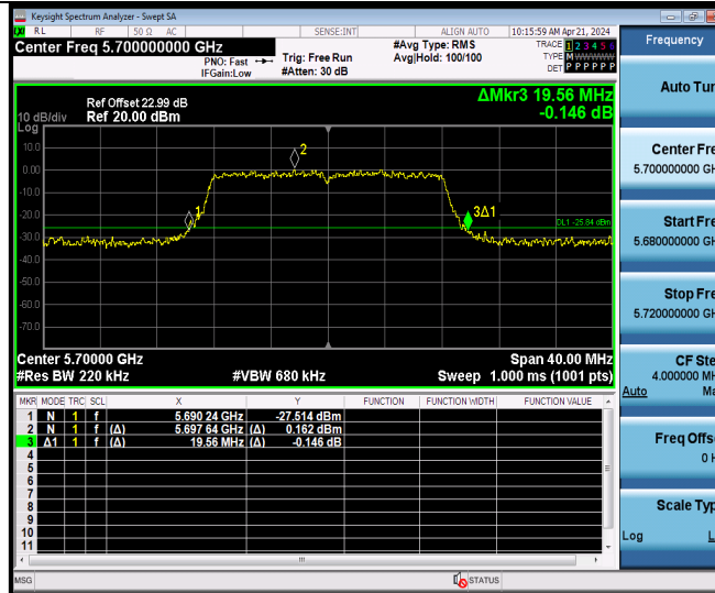
11A-CDD Ant9 5700
