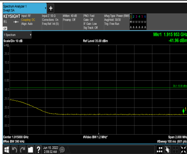
Band25-20MHz-16QAM-26590-1RB#0
