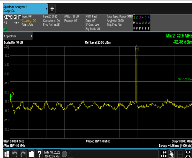
Band12-1.4MHz-QPSK-23017-1RB#0-Range1:30~1000MHz
