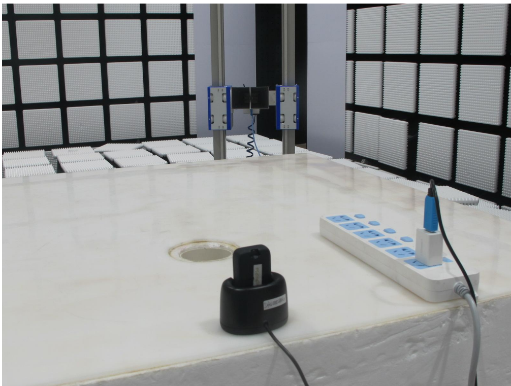
RE_1GHz-18GHz
