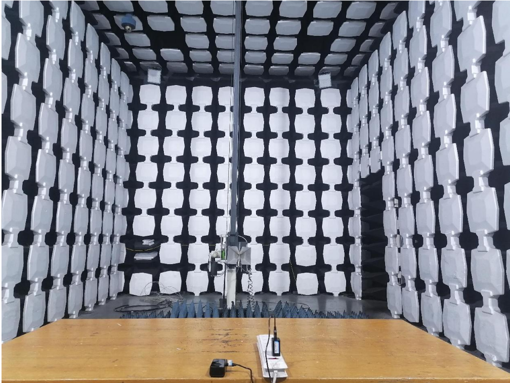
RE_1GHz-18GHz
