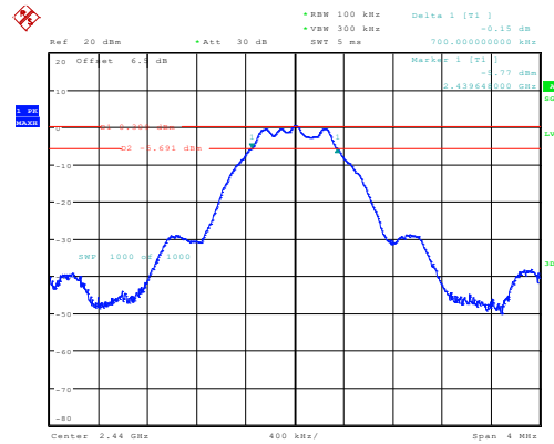
Middle 0.700MHz
