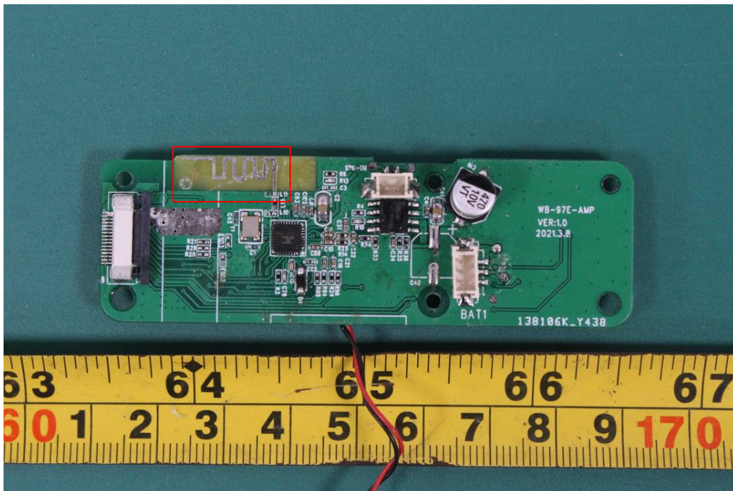
Antenna
