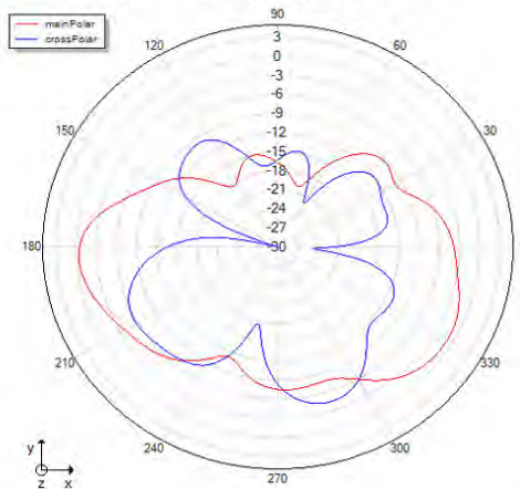
Theta=90 freq=2428MHz
