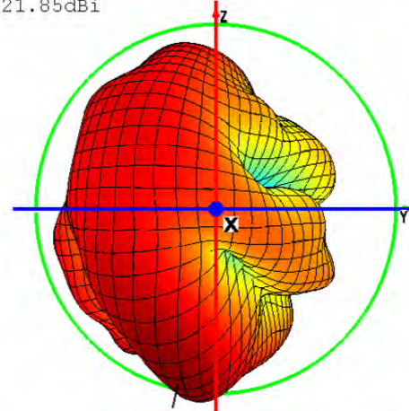
Theta=90 freq=2428MHz
