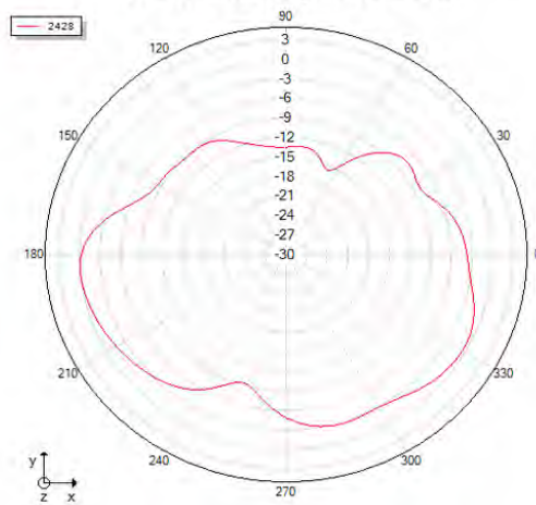
Theta=90 freq=2428MHz
